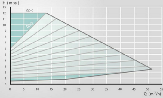
ASP 80/12 360 İNV
